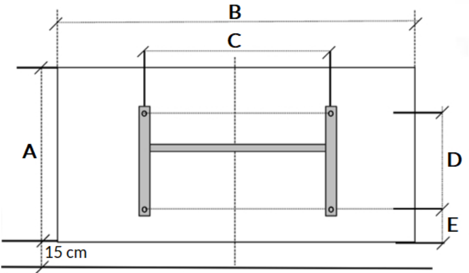
Ophangbeugel achterkant
